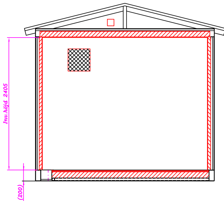
Snitt B-B
