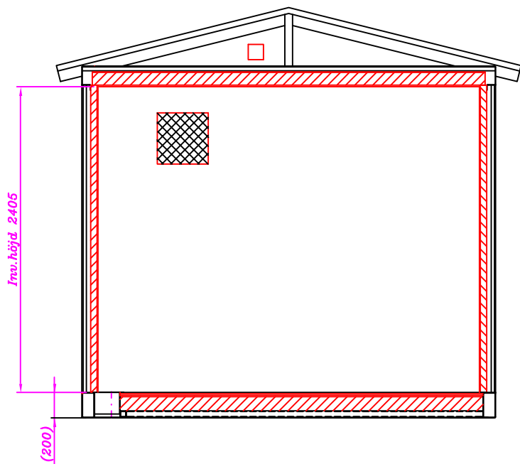
Snitt B-B
